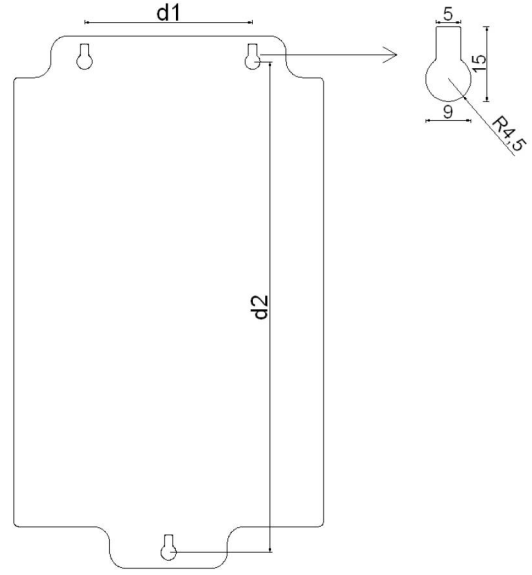
Şekil 2.2 Montaj Delikleri
